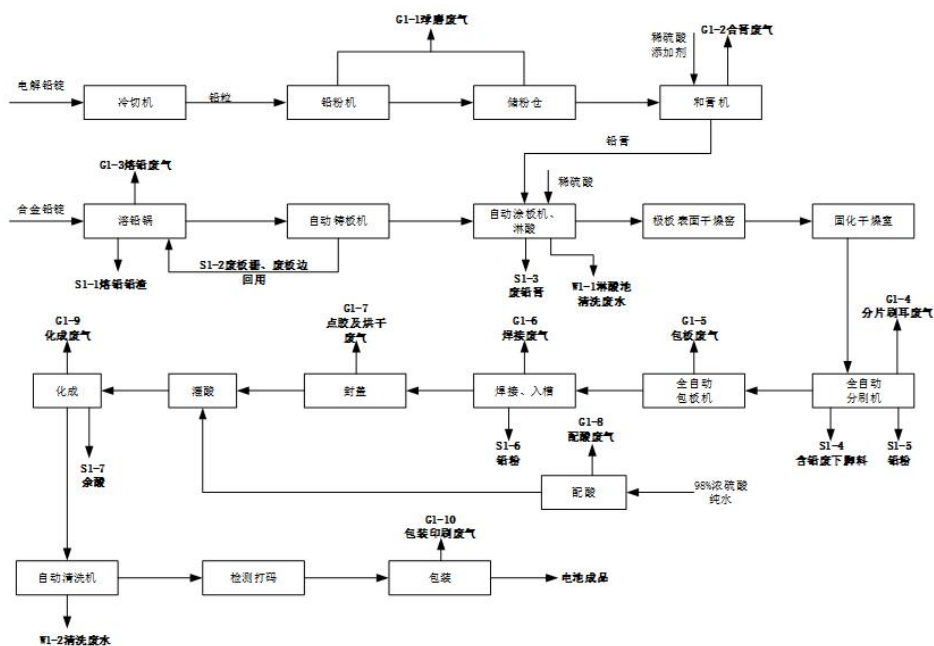
图2.3-4 中密电池生产工艺流程及产污环节图
