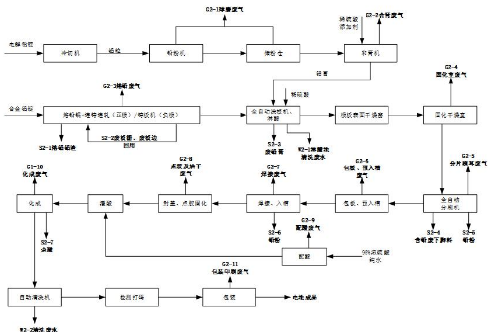
图2.3-5 小密电池生产工艺流程及产污环节图
